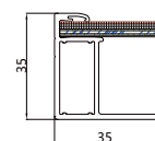
断面図 A-A
